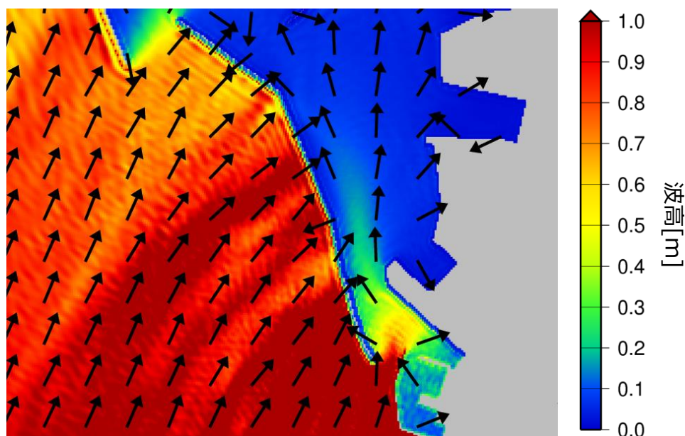
図：洋上風力設計支援に用いる波高分布の解析例
